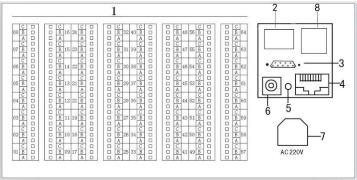
1. 信号输入(测量模组装置安装插槽)
