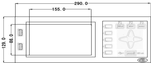
外形尺寸：129×290×300mm(高×宽×深)
